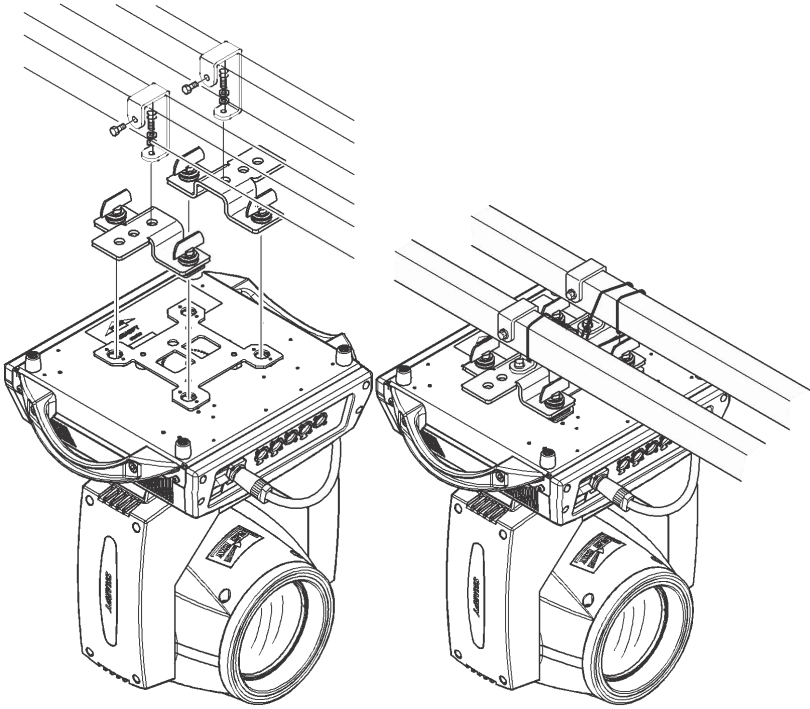
图 2 倒挂灯具示意图
